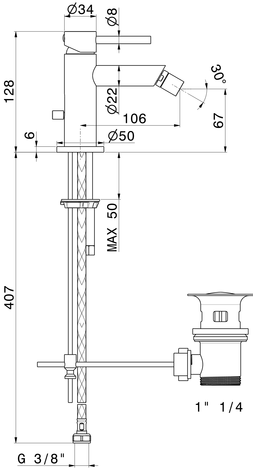
MINI-X PRO '61326'
